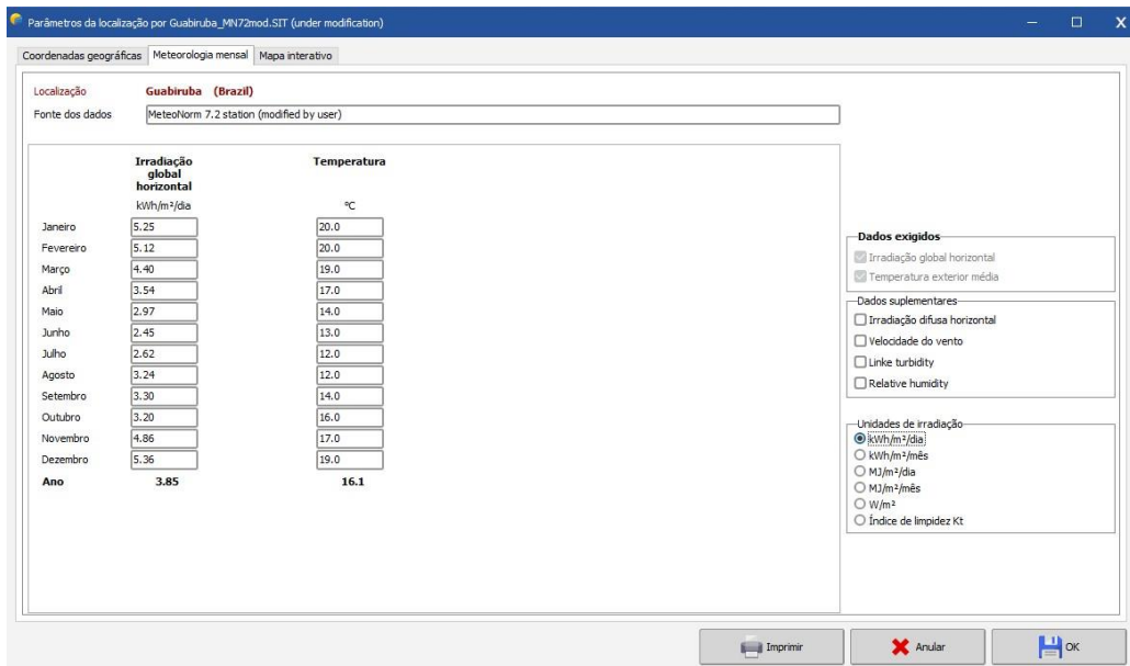
Figura 5. Inserção dos dados de irradiação e temperatura para a localidade de Guabiruba/SC (PVsyst, 2020).
