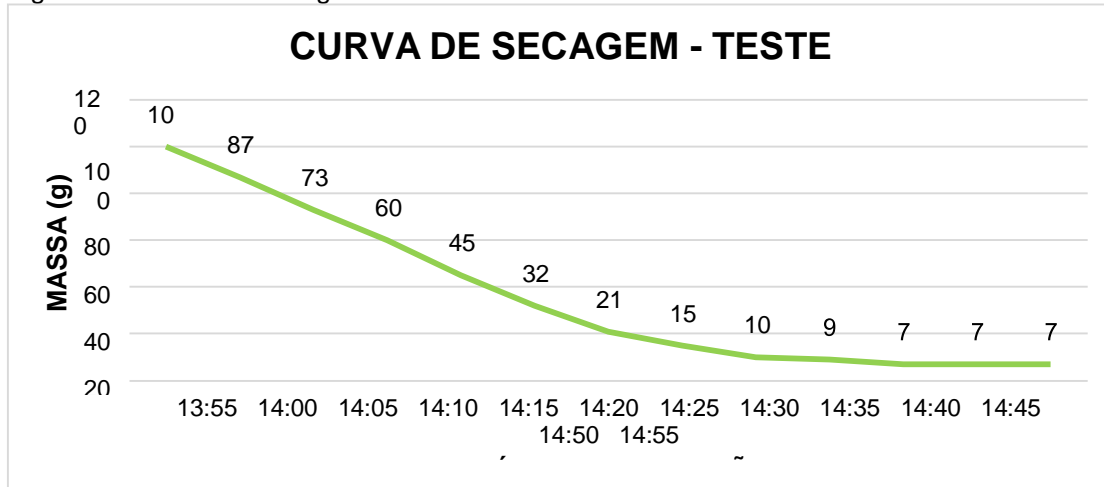
Figura 08 – curva de secagem do lodo – teste 02.
