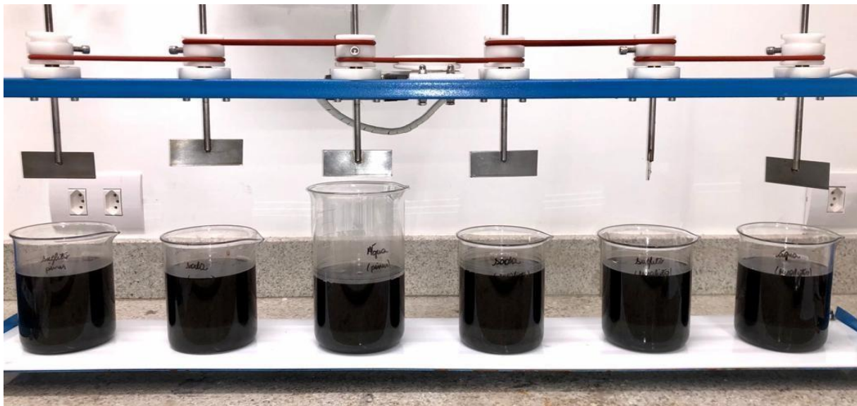
Figura 7 - Amostras de efluente preparadas para o ensaio no equipamento Jar test
